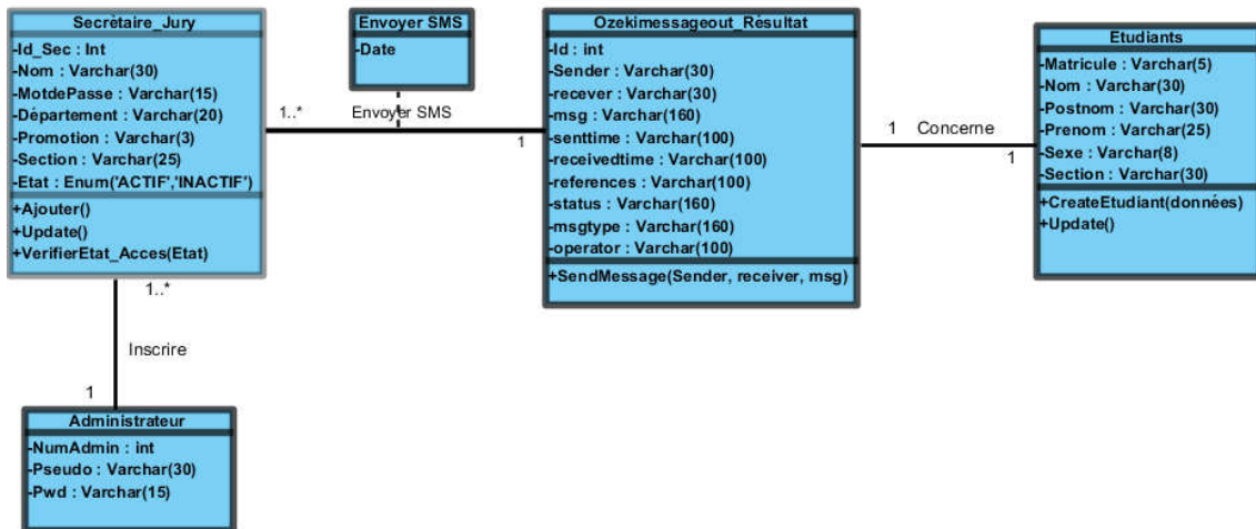
Fig. 2. Diagramme de classe
