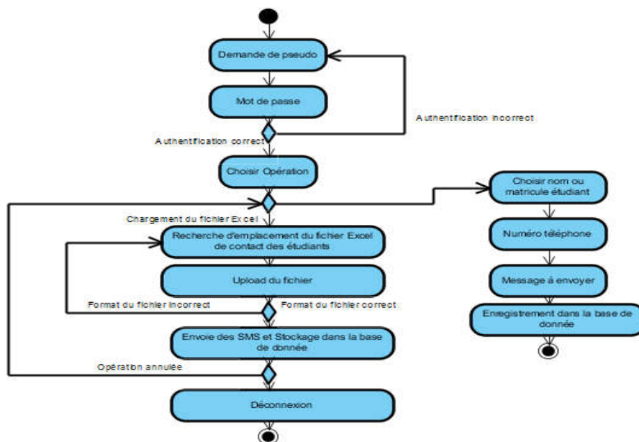
Fig. 3. Diagramme d'activité
